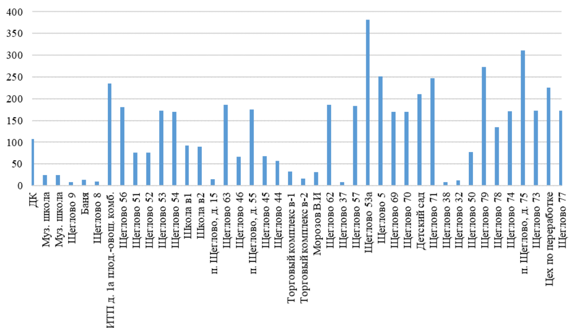
Рисунок 11.4 Средний суммарный недоотпуск теплоты потребителям котельной БМК-12,08
