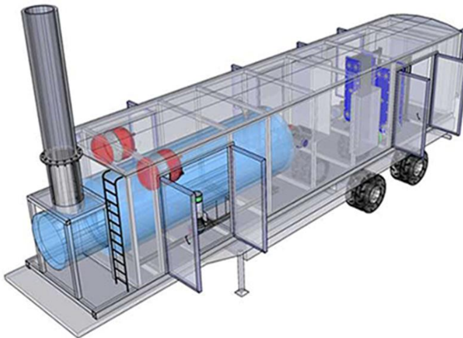
Рисунок 11.7 Схематичный вид передвижной котельной установки
