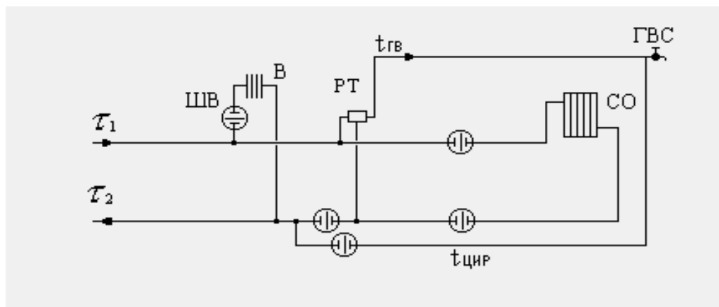
Рисунок 1.16 Схема подключения потребителей к двухтрубным системам теплоснабжения
