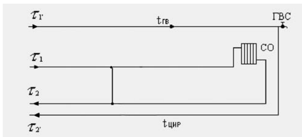
Рисунок 1.17 Схема подключения потребителей к четырехтрубным системам теплоснабжения
