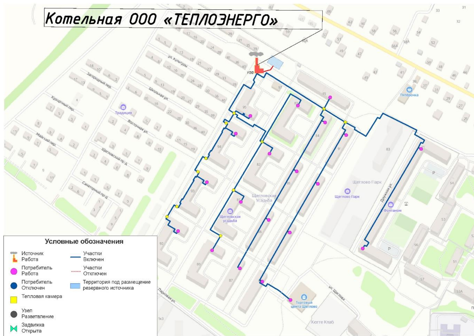
Рисунок 11.9 Предполагаемое место размещения резервного источника на БМК ООО «ТЕПЛОЭНЕРГО» пос. Щеглово
