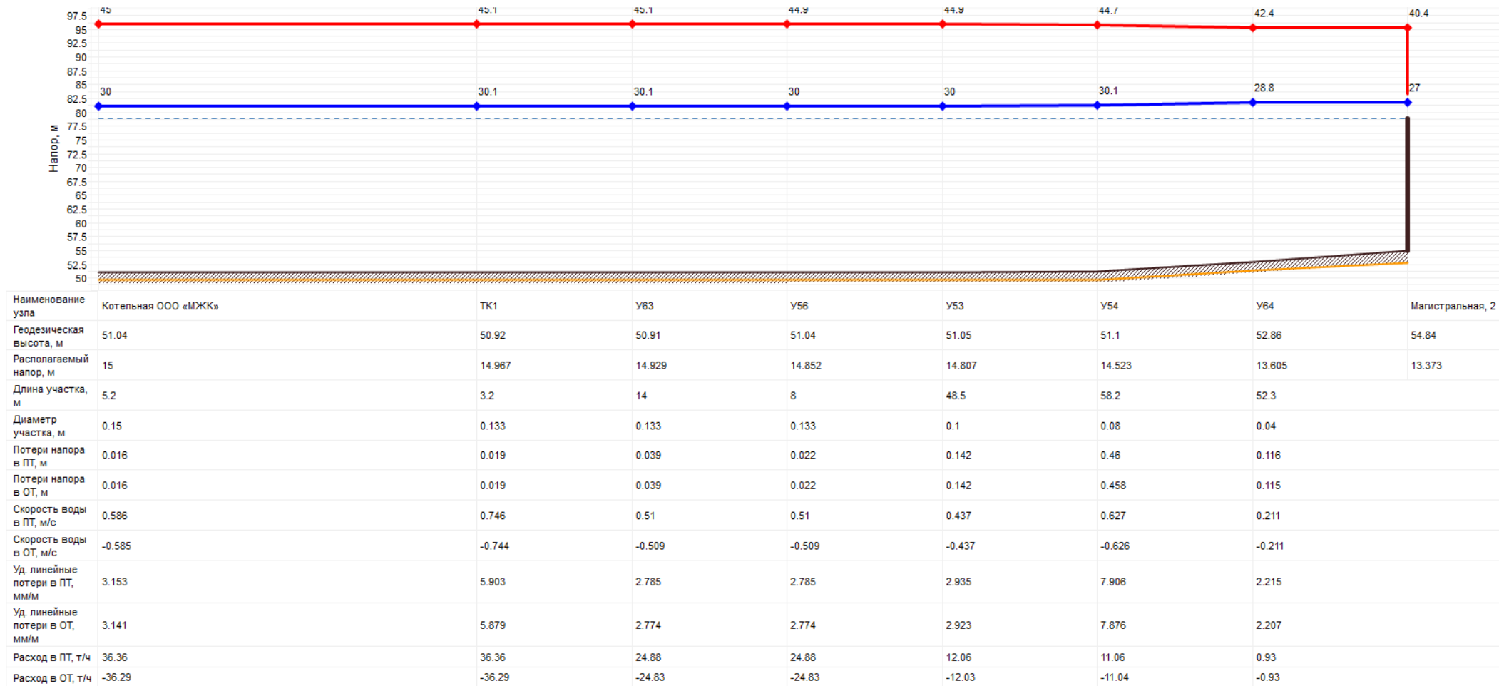
Рисунок 1.15 Пьезометрический график от котельной ООО «МЖК»
