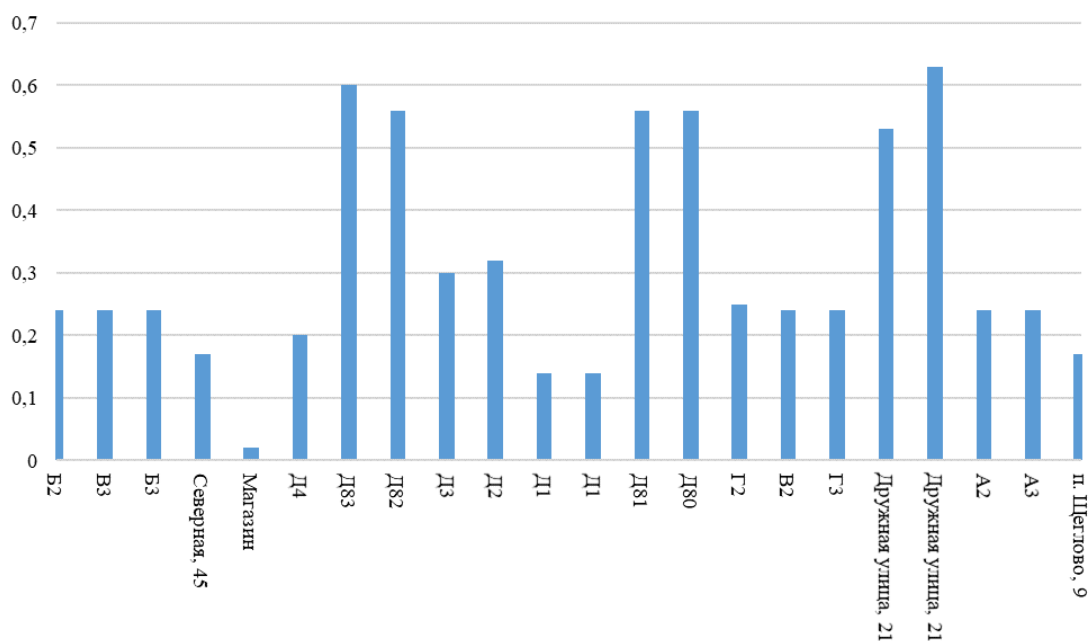
Рисунок 11.5 Средний суммарный недоотпуск теплоты потребителям котельной БМК ООО «ТЕПЛОЭНЕРГО»
