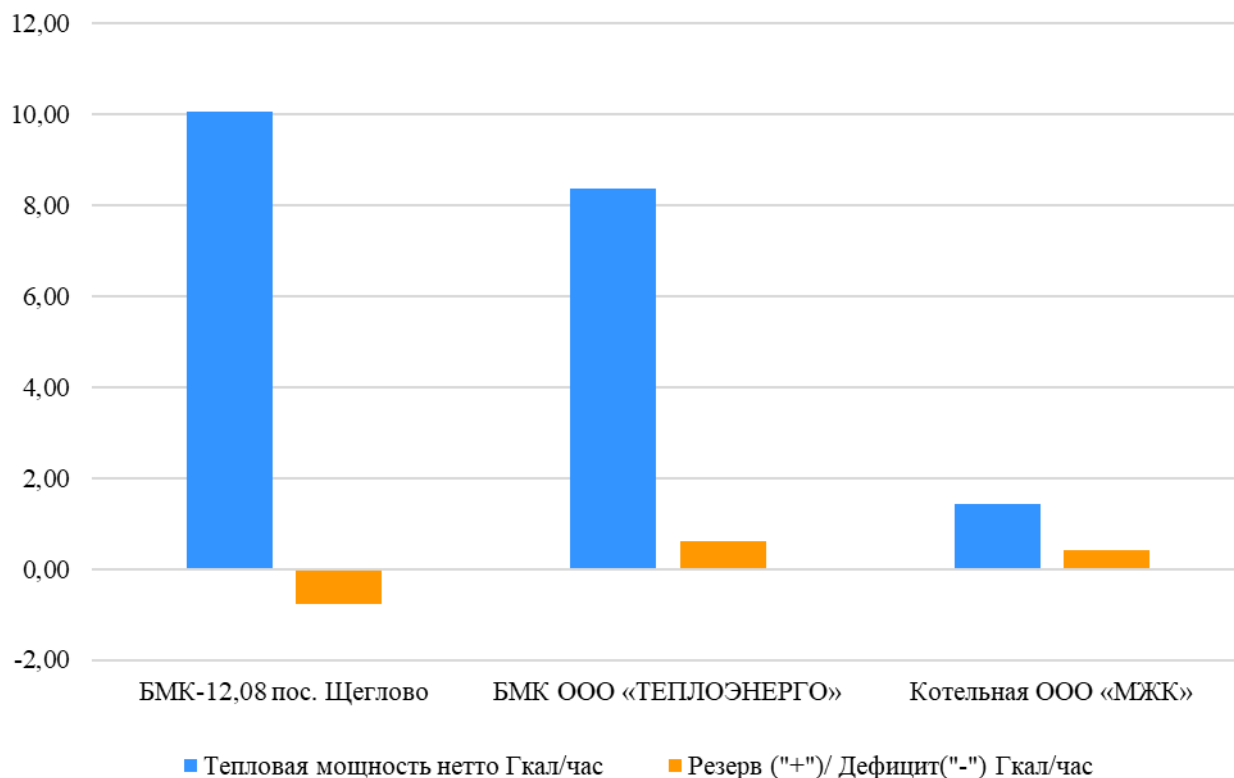
Рисунок 4.1 Балансы располагаемой тепловой мощности и резерва тепловой мощности источников
