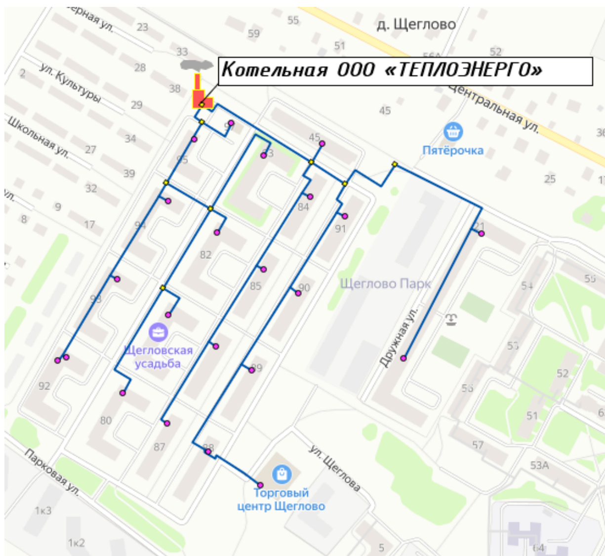
Рисунок 7. Система теплоснабжения котельной ООО «Теплоэнерго»
