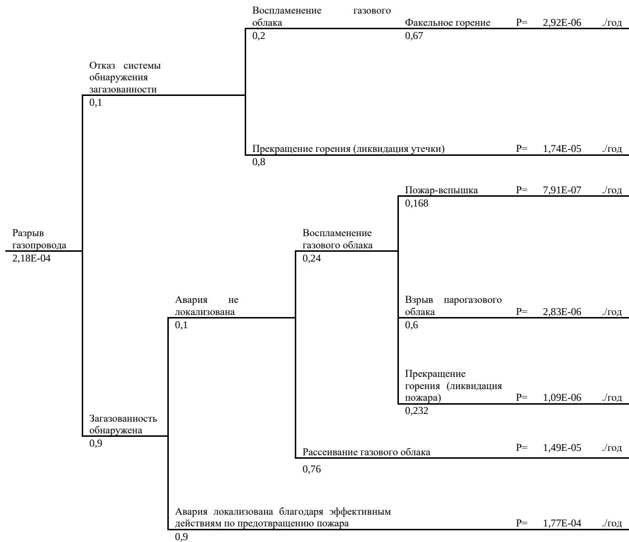
Рисунок 11. «Дерево событий» при реализации сценария C12
