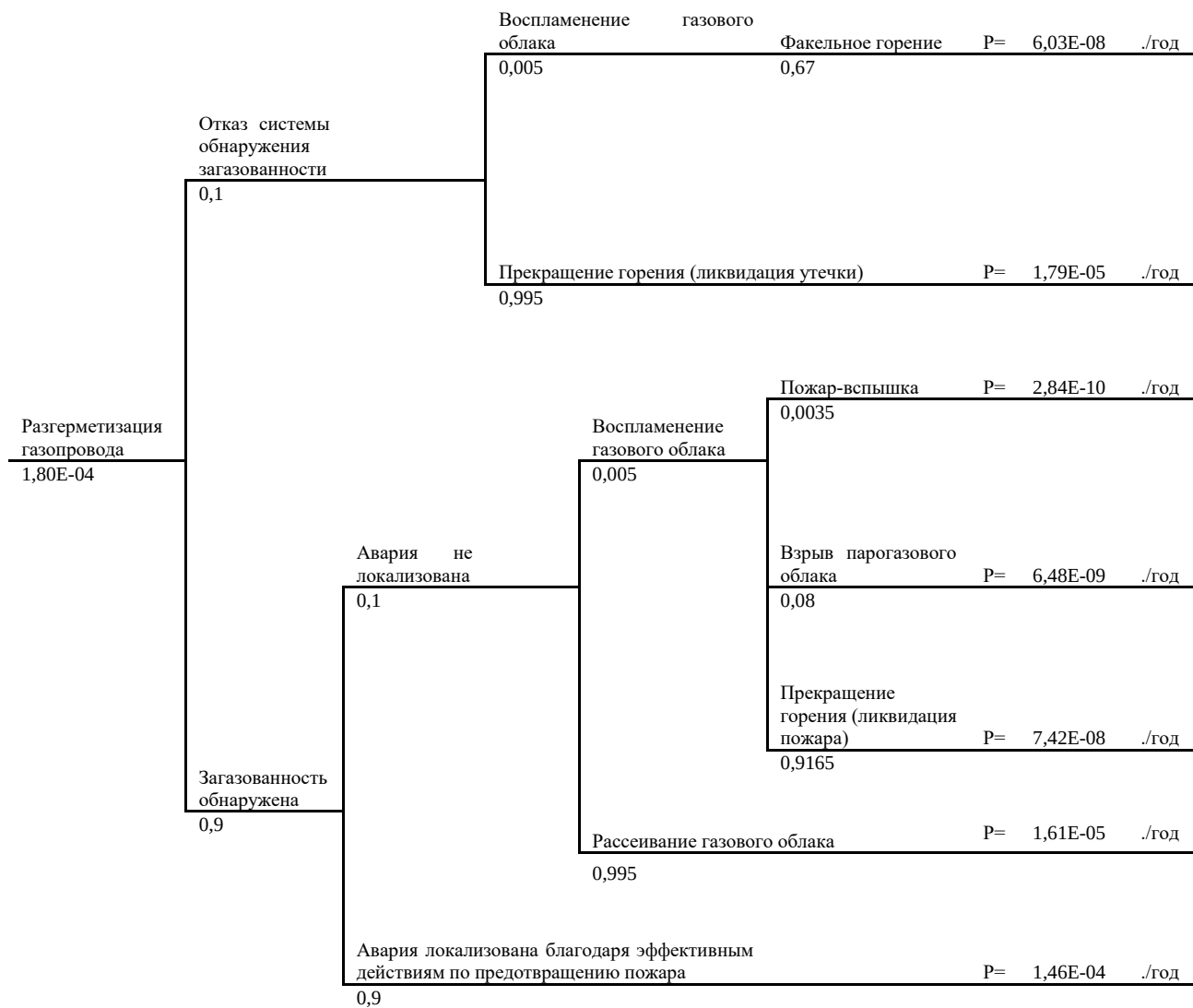
Рисунок 14. «Дерево событий» при реализации сценария С31
