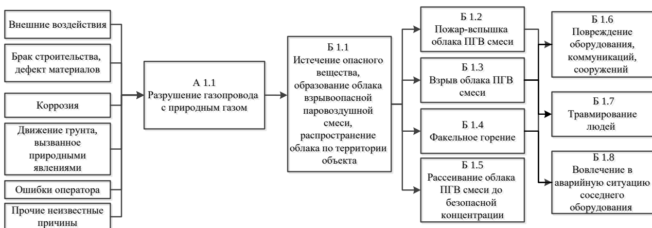
Рисунок 9.Схемы возможных сценариев возникновения и развития аварий при реализации сценария С1, С2, С3, С4, С5
