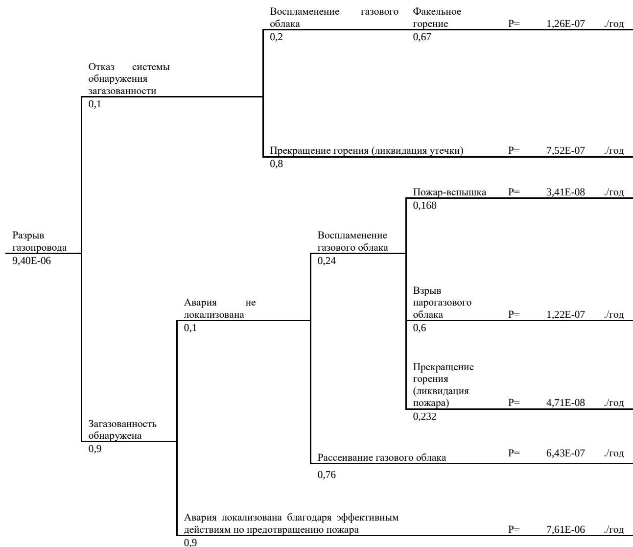
Рисунок 17. «Дерево событий» при реализации сценария С42
