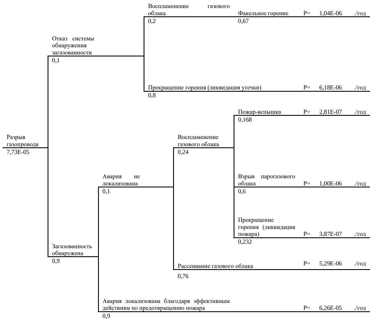
Рисунок 15. «Дерево событий» при реализации сценария С32
