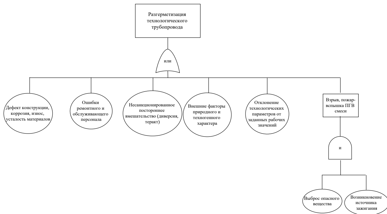
Рисунок 20. «Дерево отказов» анализа причин аварийной ситуации и ее проявления при реализации сценариев разгерметизации технологических трубопроводов
