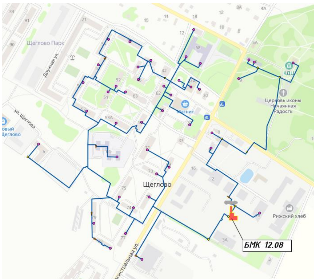
Рисунок 6. Система теплоснабжения котельной БМК 12.08
