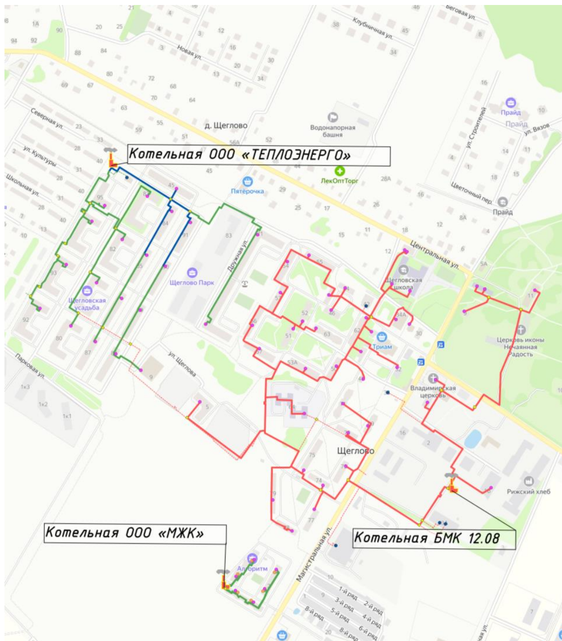
Рисунок 3.Схема систем теплоснабжения Щегловского сельского поселения
