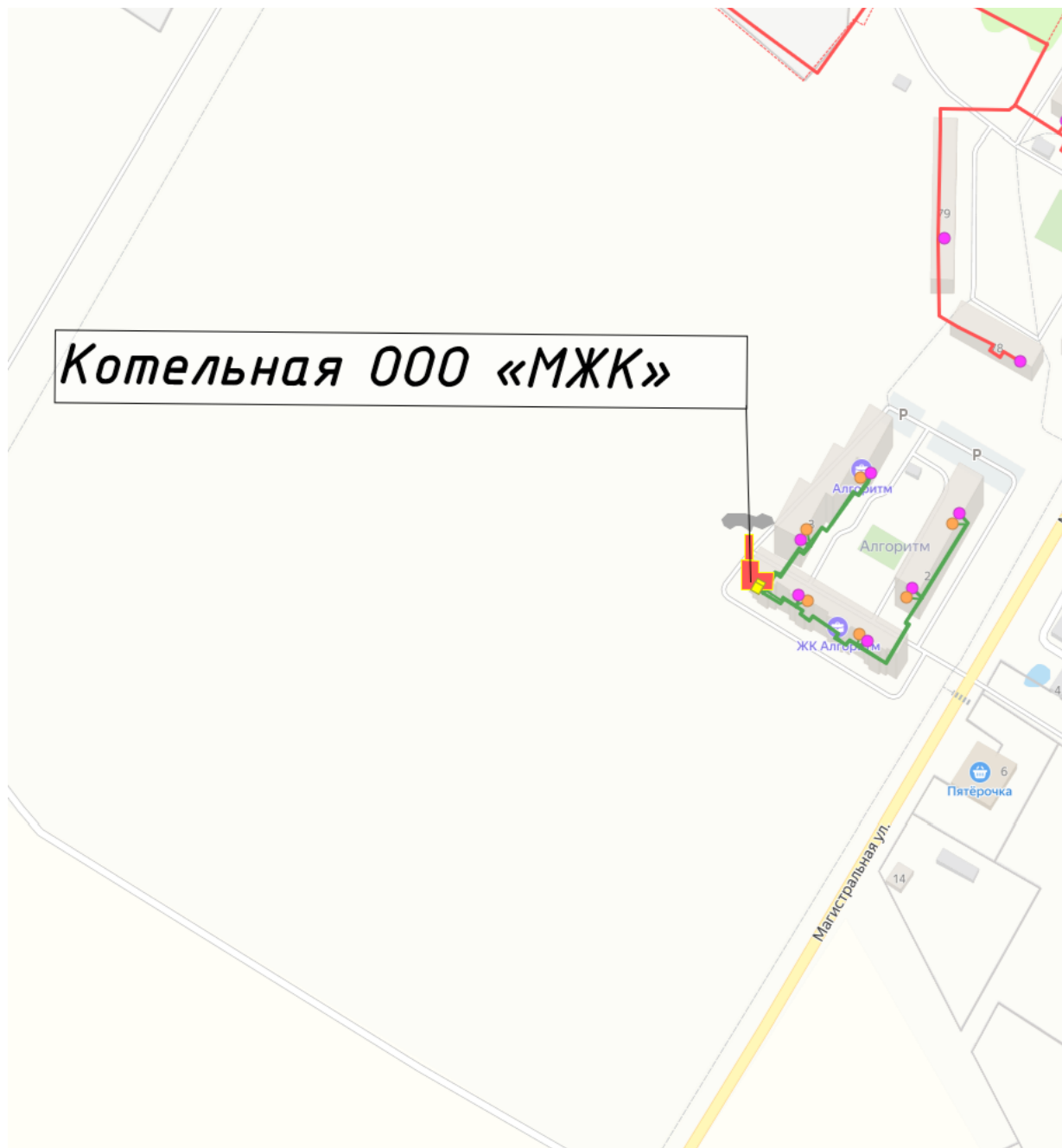
Рисунок 8. Система теплоснабжения котельной ООО «МЖК»
