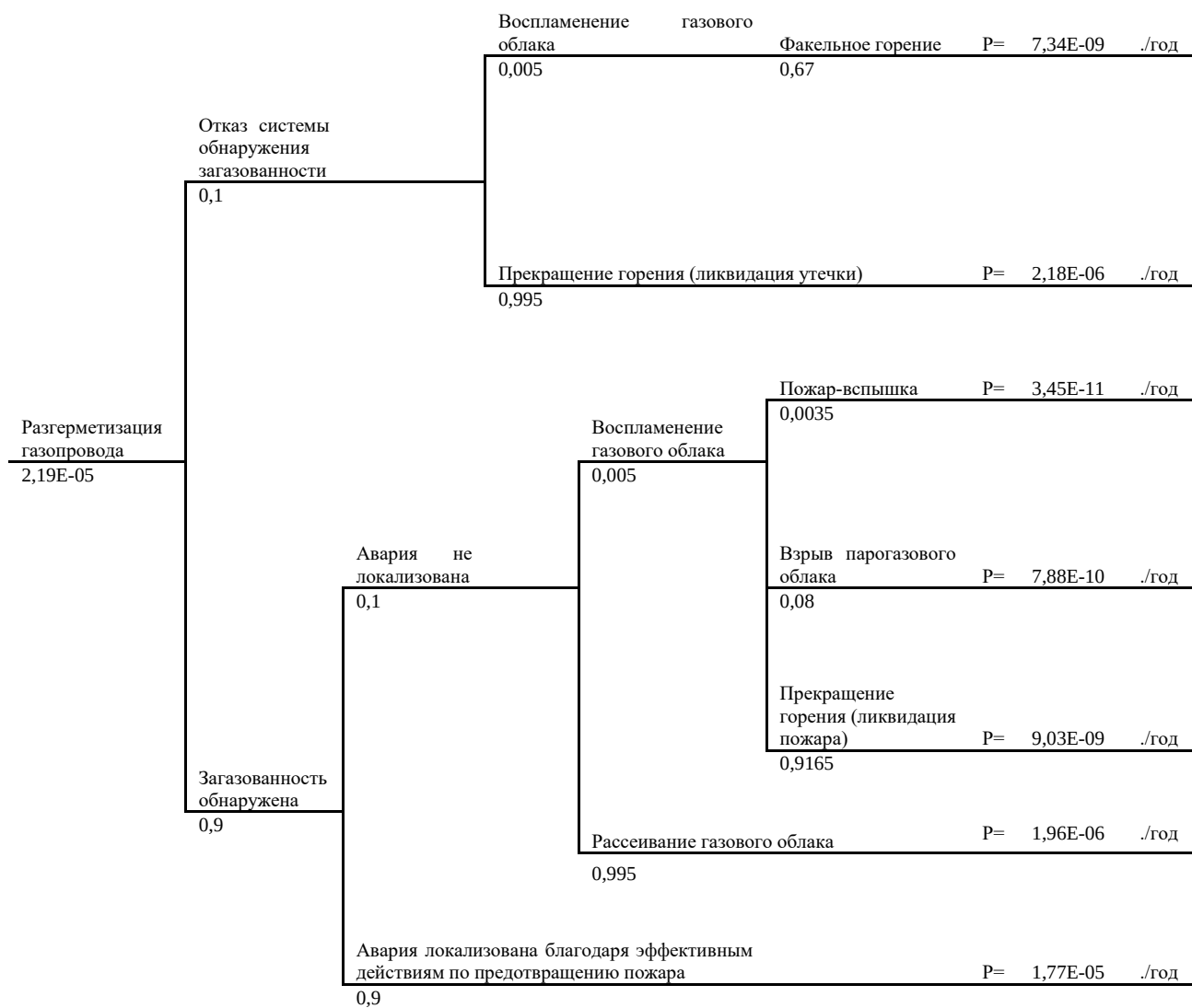
Рисунок 16. «Дерево событий» при реализации сценария С41
