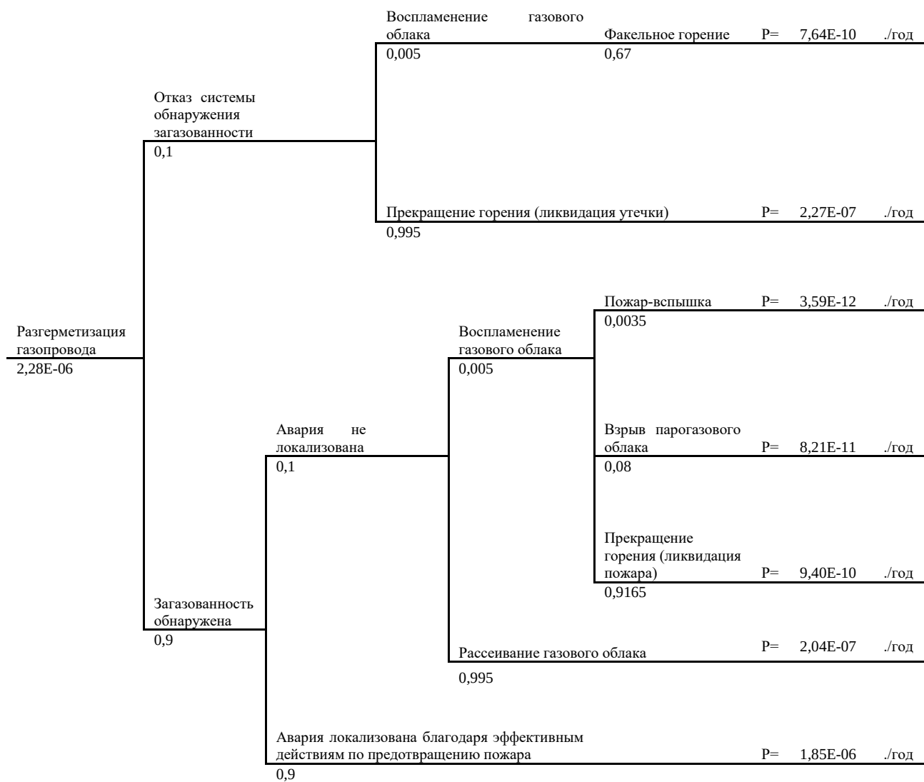
Рисунок 18. «Дерево событий» при реализации сценария C51
