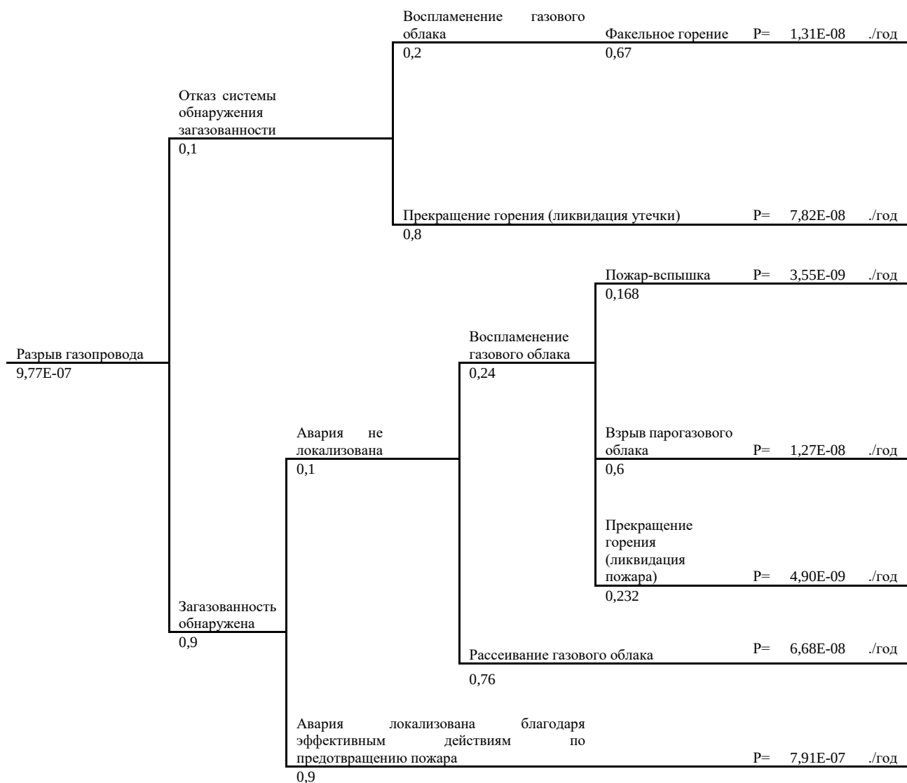
Рисунок 19. «Дерево событий» при реализации сценария C52
