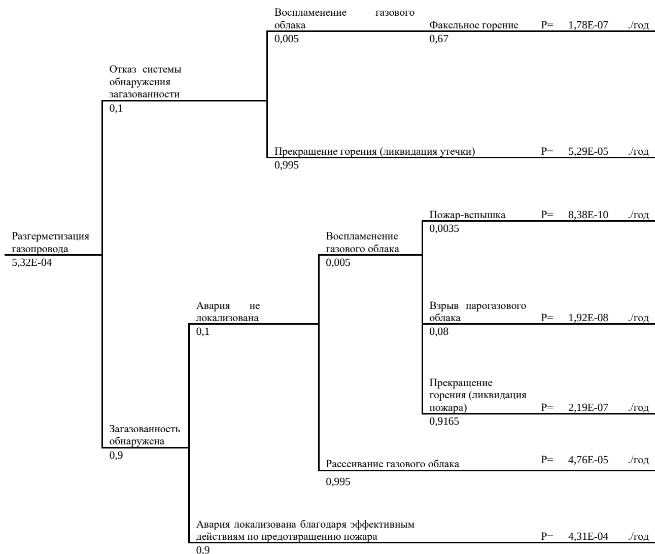
Рисунок 10. «Дерево событий» при реализации сценария C11
